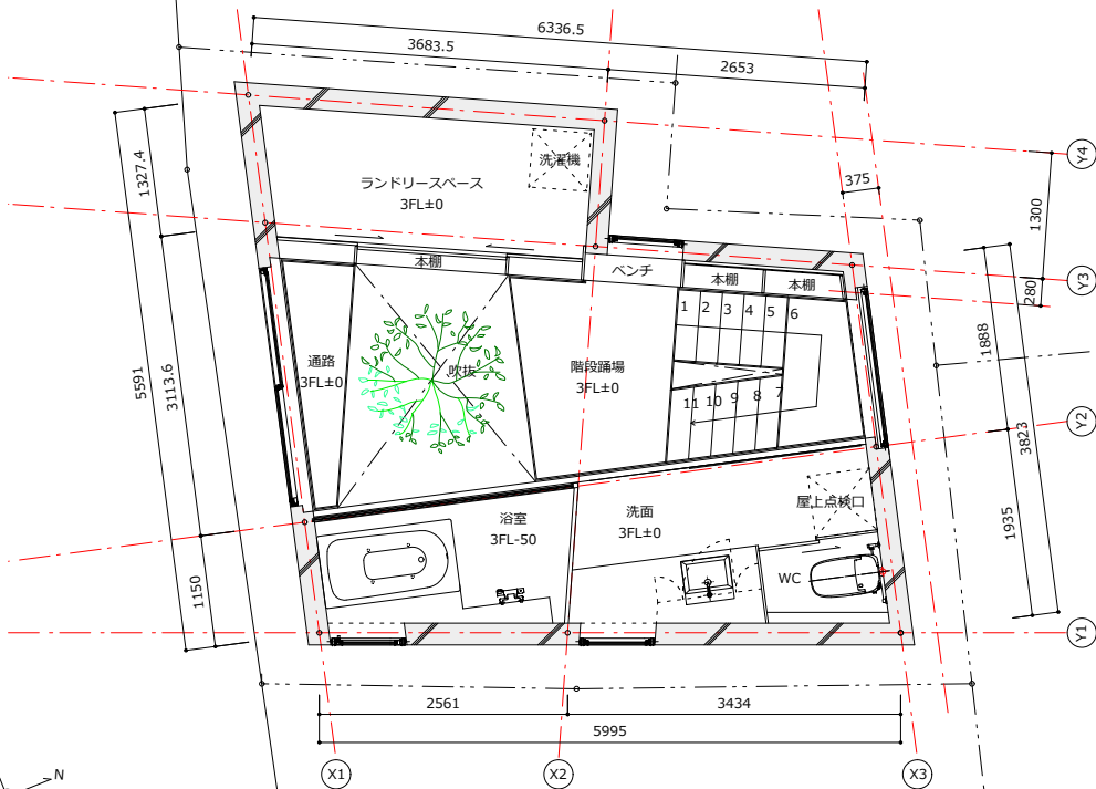
□3F平面図 S=1/100
