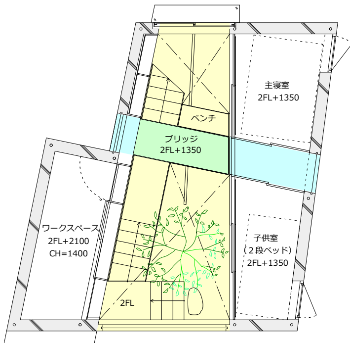
2.5F平面図
